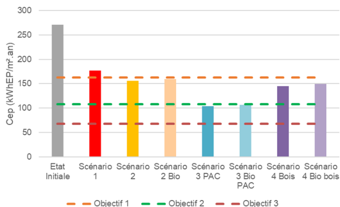
Evolution du Cep et des objectifs du Cahier des Charge
